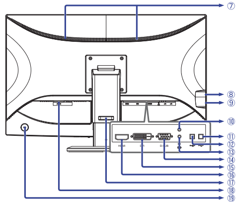
<Arrière>
