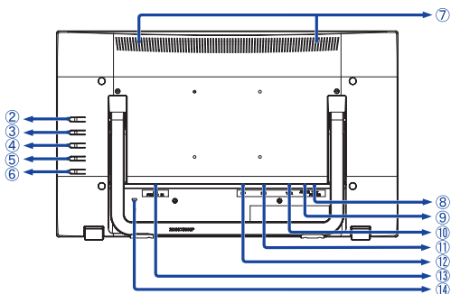
<Вид сзади>
