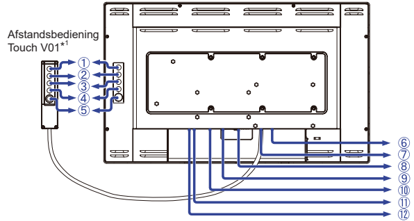
<Achterkant>
